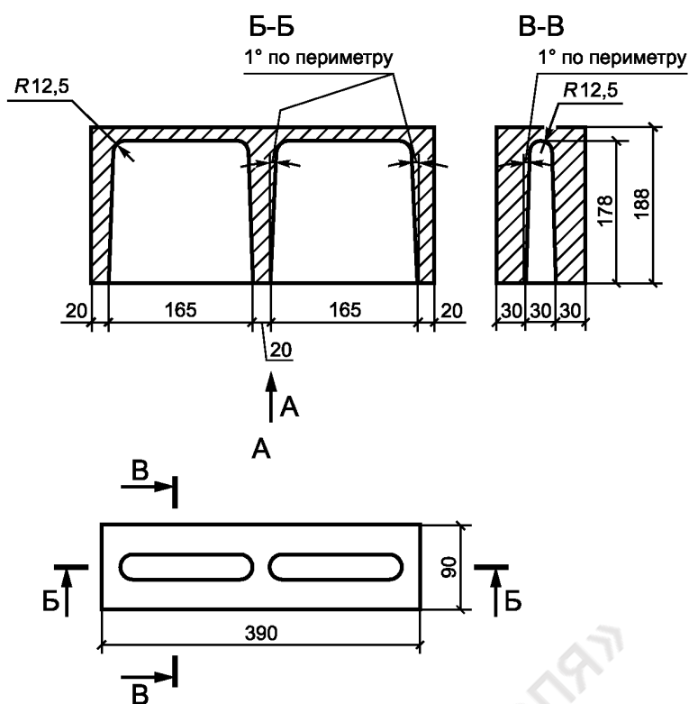
Рисунок А.17 — Камень стеновой рядовой (продольная половинка)
